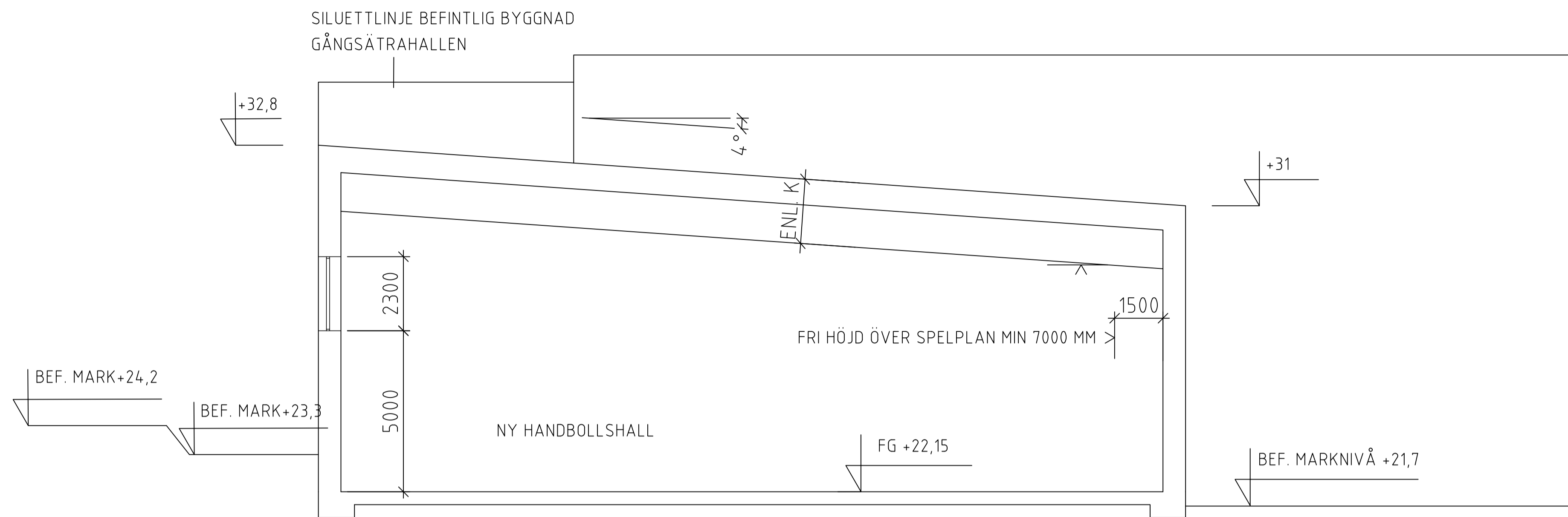
SEKTION A-A ALLA HÖJDER I RH 2000
